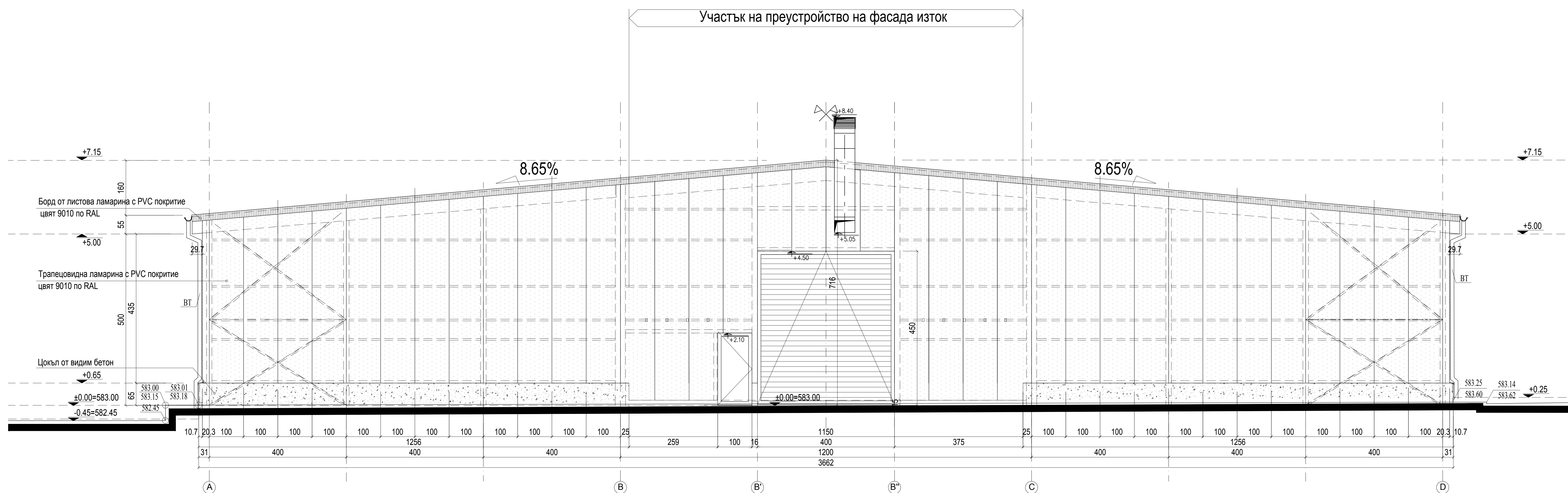
Фасада Изток М 1:50
