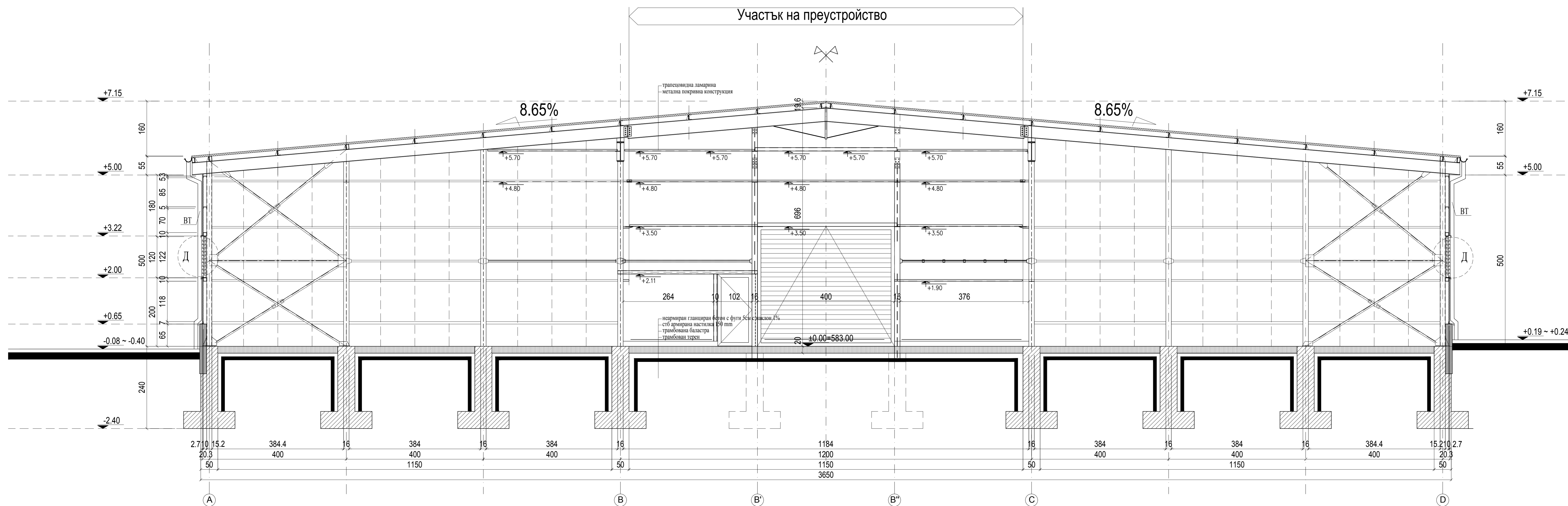
Разрез G1-G1
